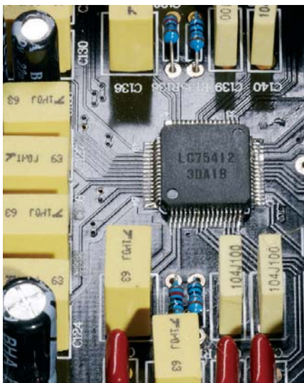
Eingangssektion mit hochwertigen Folien-Kondensatoren im Signalweg
